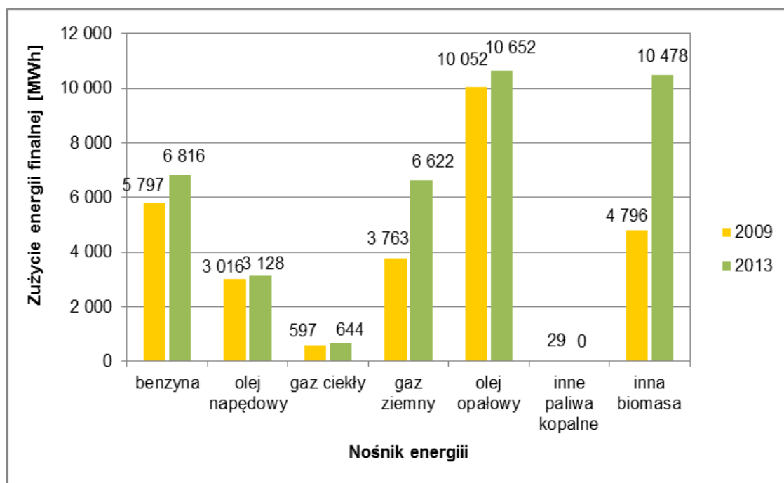
Wykres nr 16: Struktura finalnego zużycia energii w roku bazowym i kontrolnym w podziale na pozostałe nośniki [MWh]
