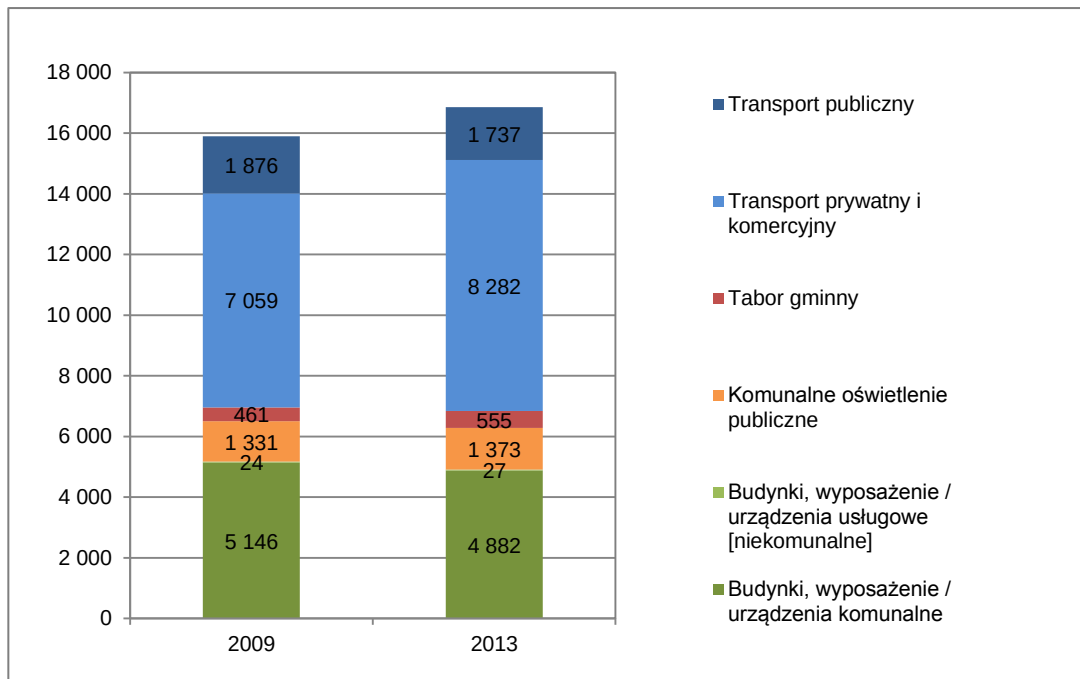
Wykres nr 14: Struktura finalnego zużycia energii w roku bazowym i kontrolnym w odniesieniu do podsektorów działalności, z wyłączeniem budynków mieszkalnych [MWh]
