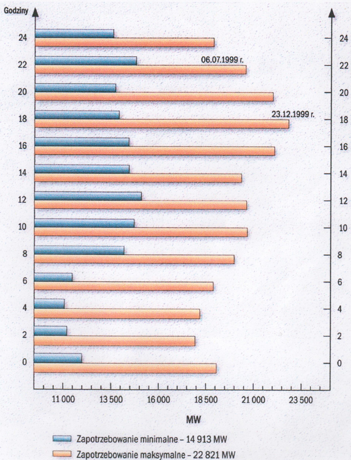
Wykresy dobowego zapotrzebowania na moc dla dnia o maksymalnym i minimalnym zapotrzebowaniu w szczycie wieczornym w 1999r.
